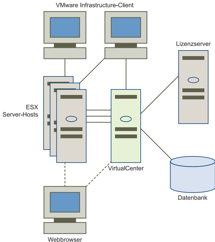
Abbildung 1-1. VMware Infrastructure-Komponenten
