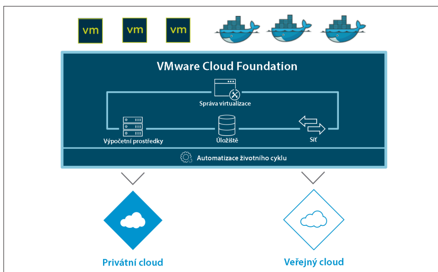
Obrázek 1: Softwarová architektura řešení VMware Cloud Foundation
