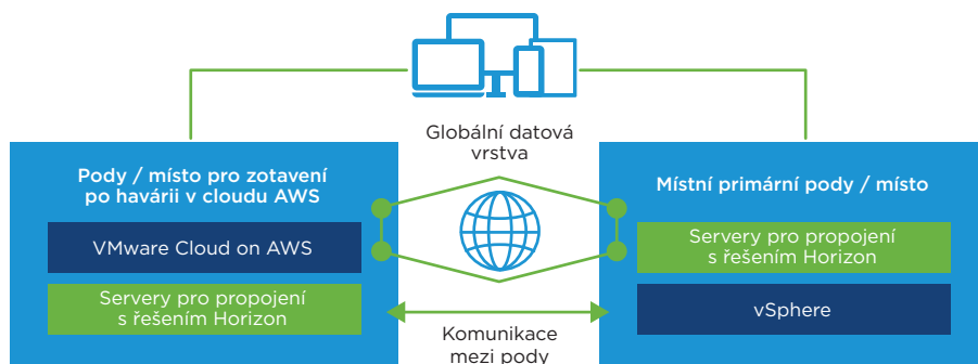
Obrázek 2: Architekturu CPA (Cloud Pod Architecture) řešení Horizon je možné roztáhnout mezi místním prostředím a cloudem AWS
