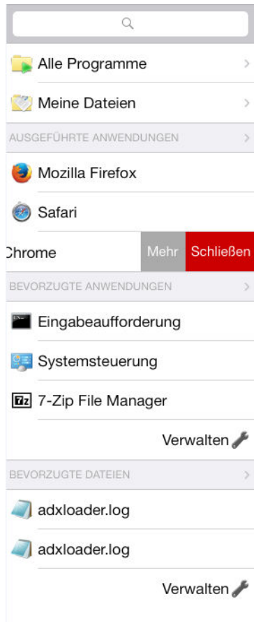
Abbildung 4-1. Unity Touch-Sidebar
