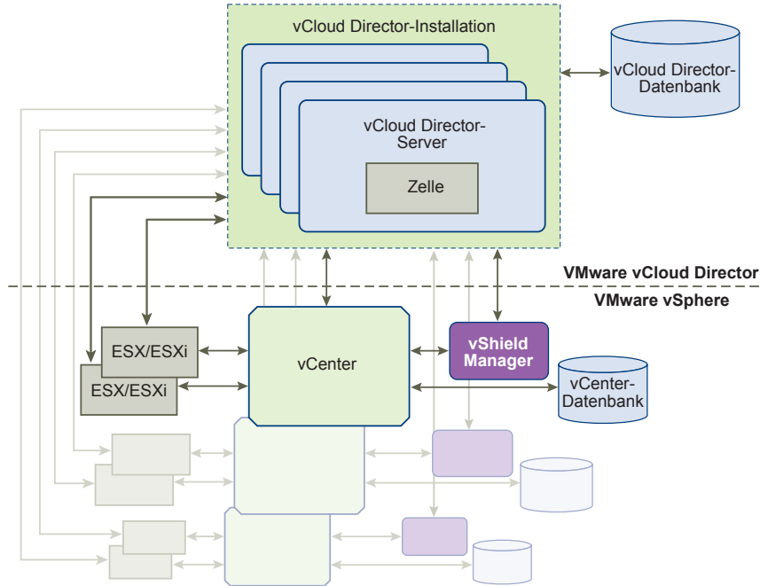
Abbildung 1-1. vCloud Director-Architekturdiagramm
