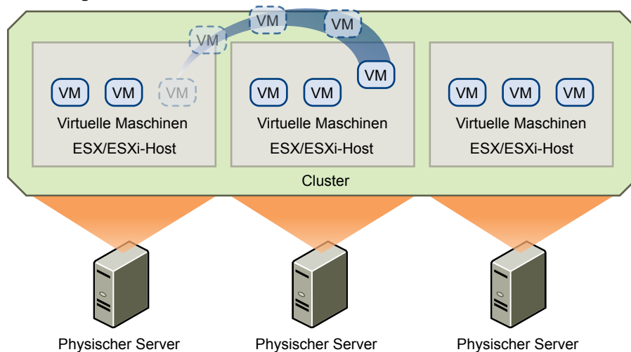
Abbildung 6. VMware DRS
