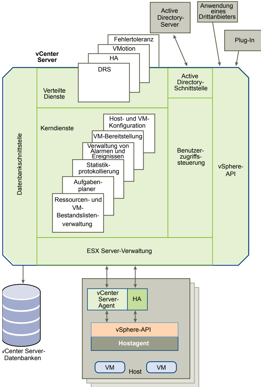
Abbildung 13. vCenter Server-Komponenten
