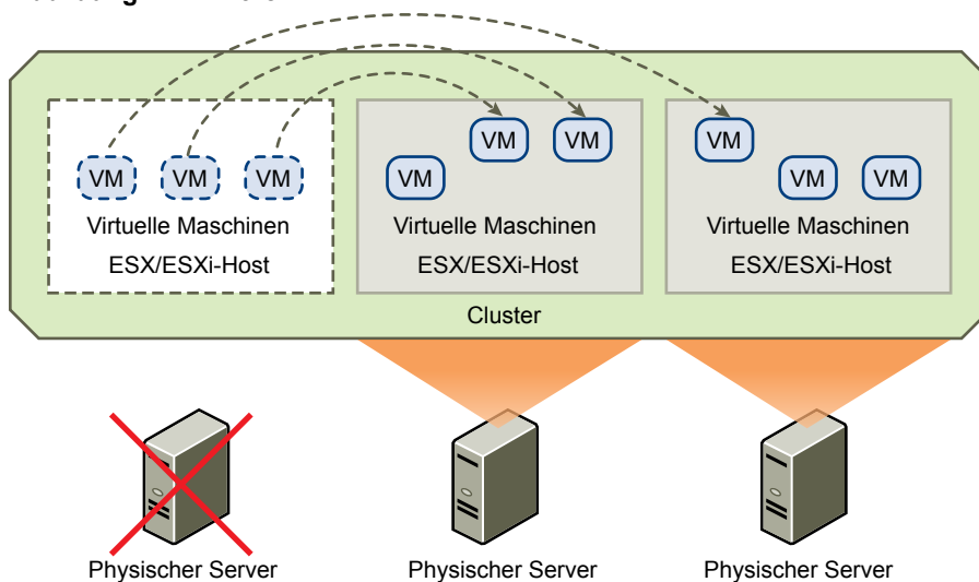
Abbildung 7. VMware HA
