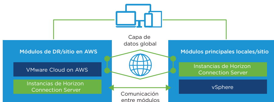
Figura 2: La arquitectura CPA de Horizon puede abarcar implementaciones locales y AWS
