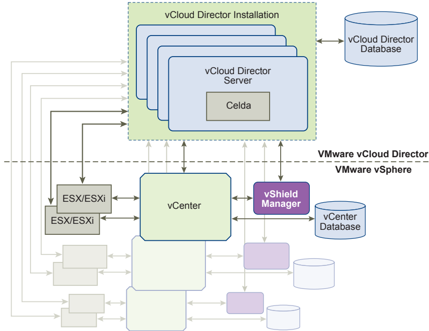
Figura 1-1. Diagrama de la arquitectura de vCloud Director
