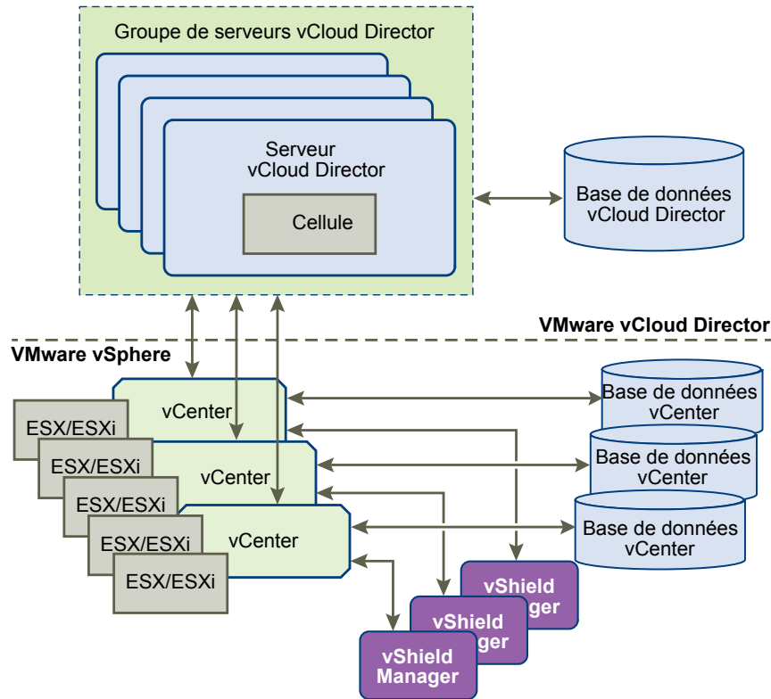
Figure 1-1. Diagramme de l'architecture de vCloud Director
