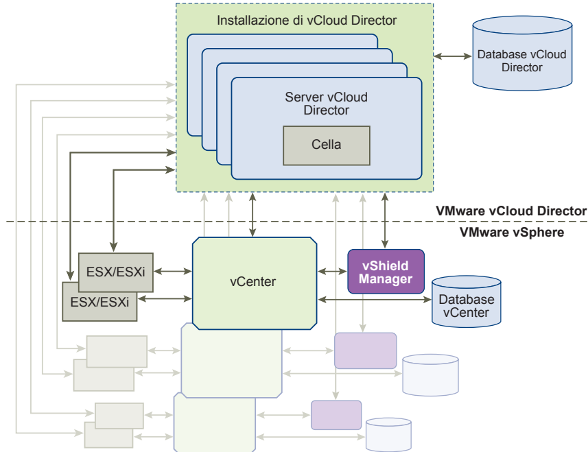
Figura 1-1. Diagramma dell'architettura di vCloud Director
