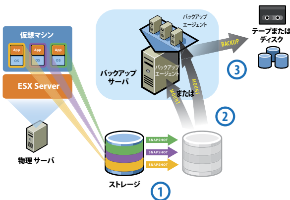
図 1: VMware Consolidated Backup により、仮想マシンのオフホストバックアップが可能
