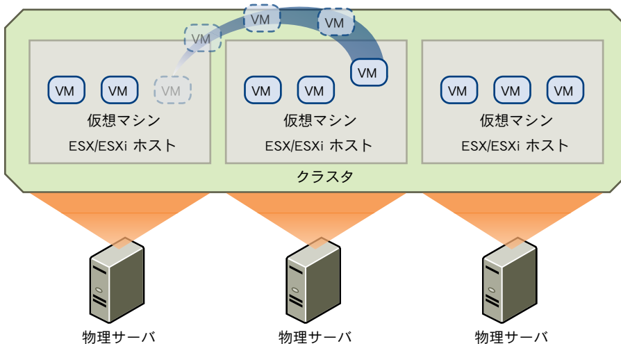
図 6. VMware DRS
