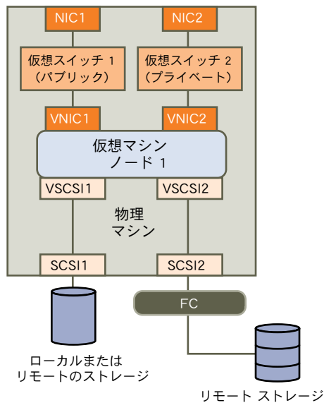
図 3-1. 最初のノードを設定した筐体間クラスター
