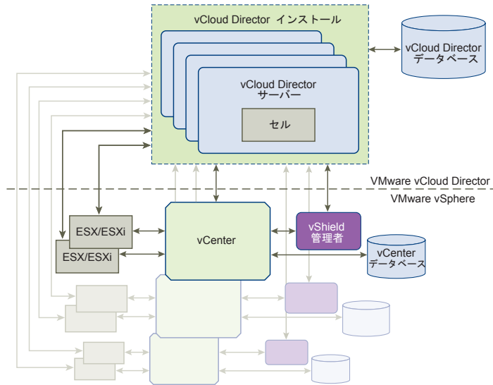
図 1-1. vCloud Director アーキテクチャ図
