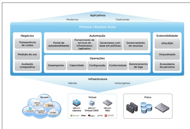
Figura 1: Componentes do vRealize Suite
