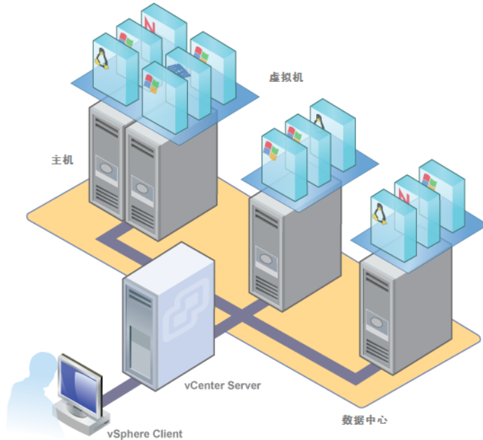
图 2 vSphere 组件
