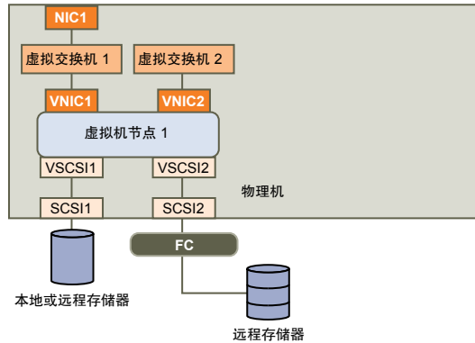
图 2-1 单节点的机箱内群集设置
