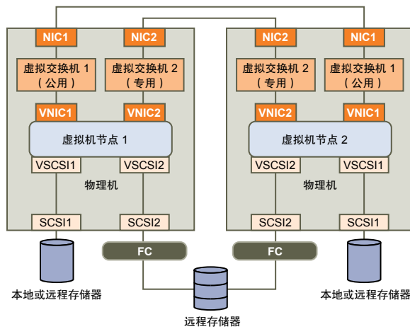
图 3-2 跨机箱的群集的完整设置
