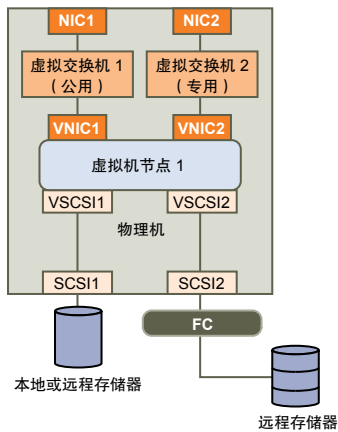
图 3-1 已设置第一个节点的跨机箱的群集
