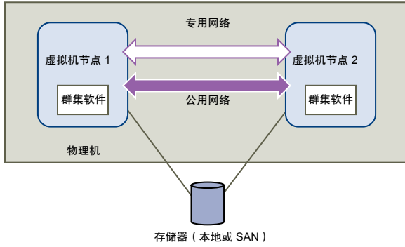
图 1-1 单个主机上群集的虚拟机
