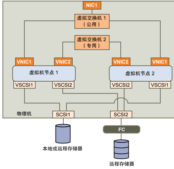
图 2-2 机箱内群集的完整设置
