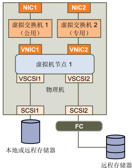
图 3-1。 设置了第一个节点的机箱间群集
